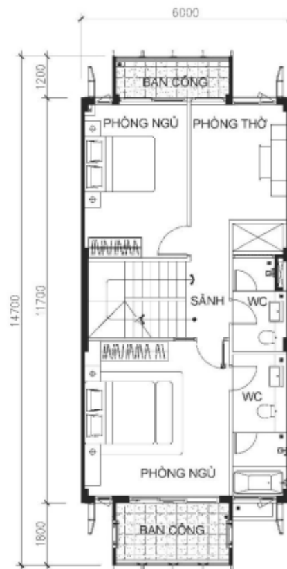
MẶT BẰNG TẦNG 3
