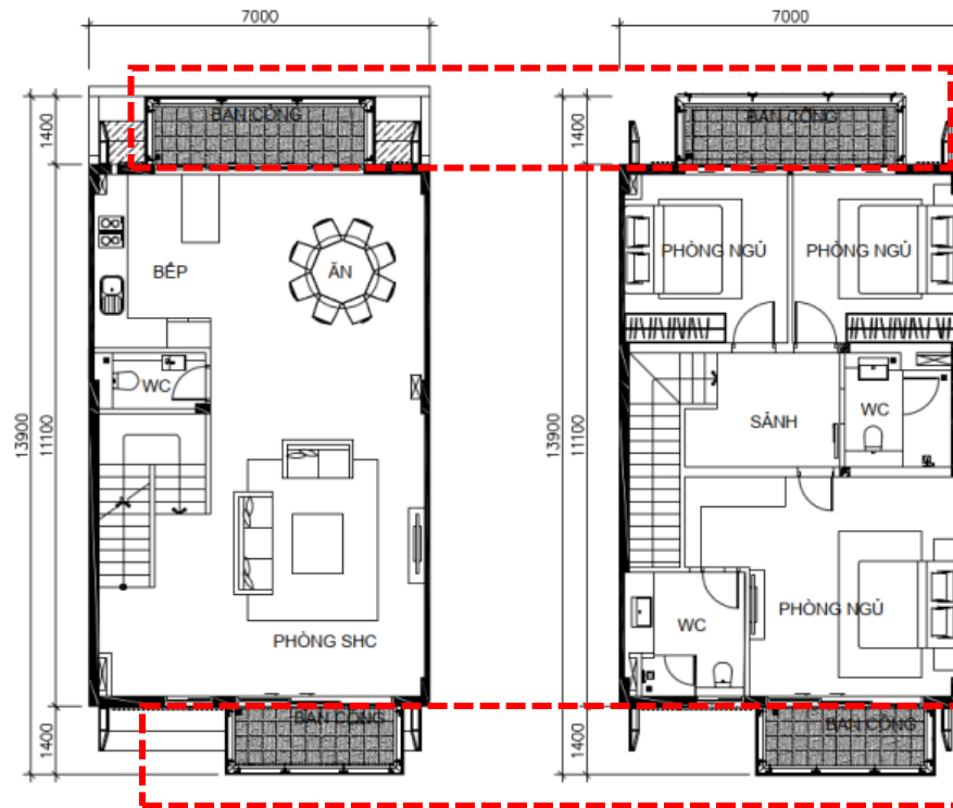
MẶT BẰNG TẦNG 3
