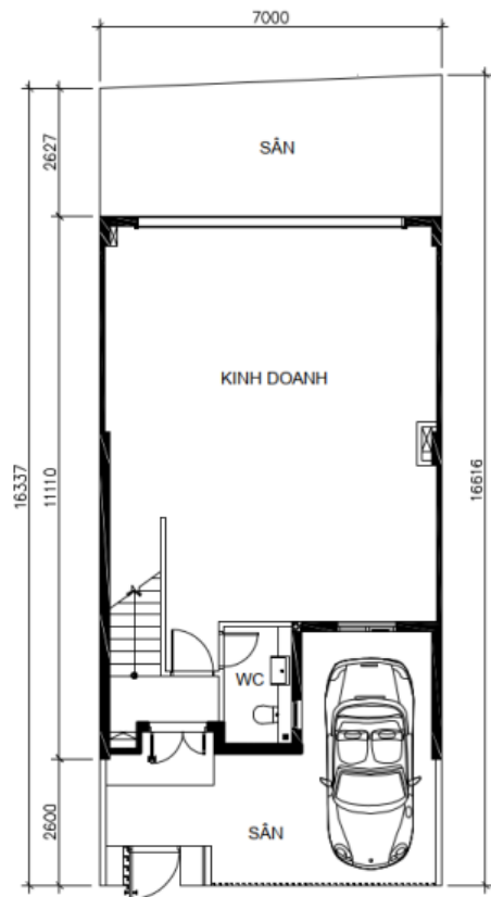
MẶT BẰNG TẦNG 1
