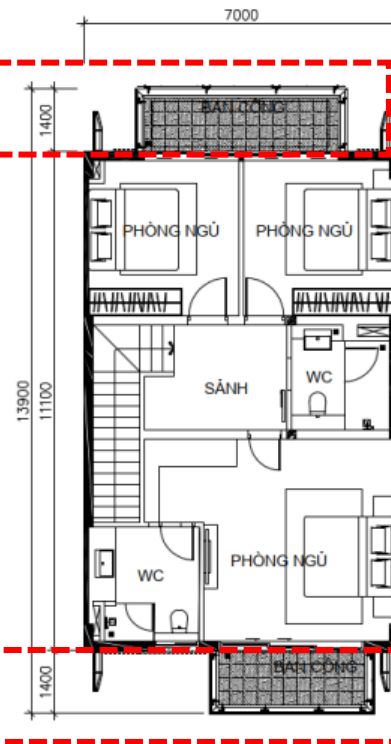
MẶT BẰNG TẦNG 4
